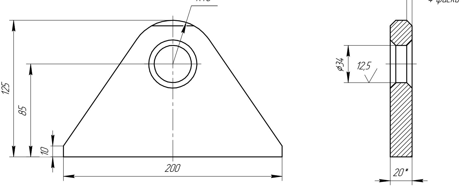
Дет. поз.13 (1:2)
