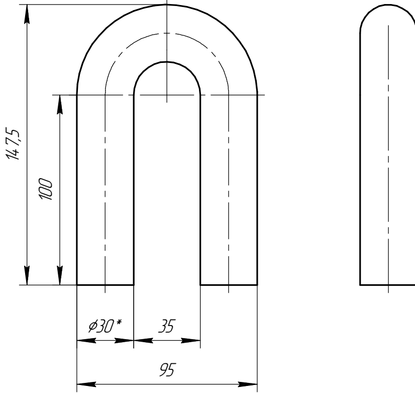
Дет. поз.7 (1:1)
