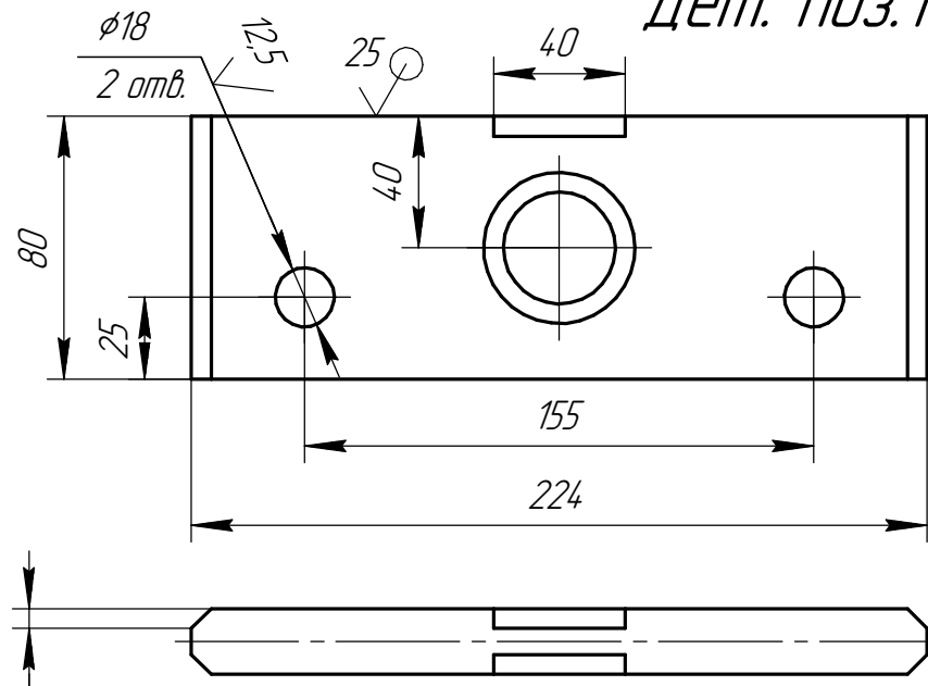
Дет. поз.11 (1:2,5)
