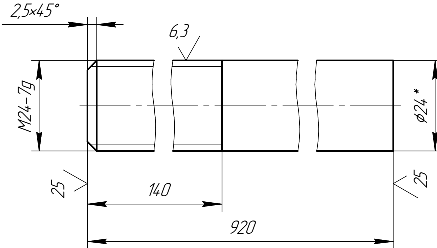
Дет. поз.13 (1:2)
