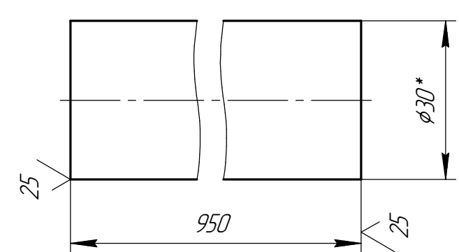
Дет. поз.12 (1:1)
