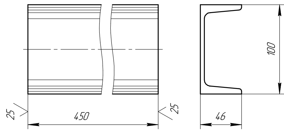
Дет. поз.5 (1:1)
