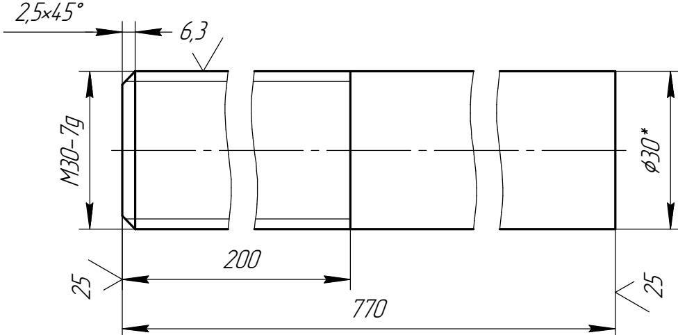
Дет. поз.7 (1:1)
