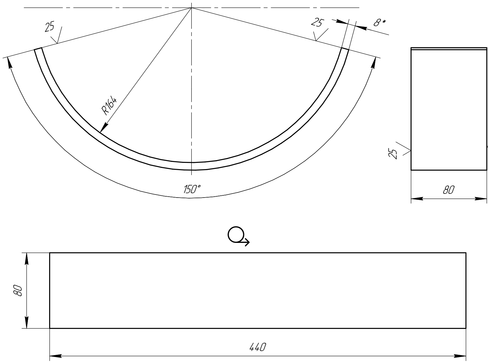
Дет. поз.3 (1:2)
