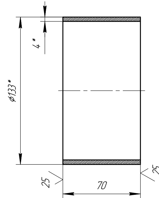
Дет. поз.9 (1:2)
