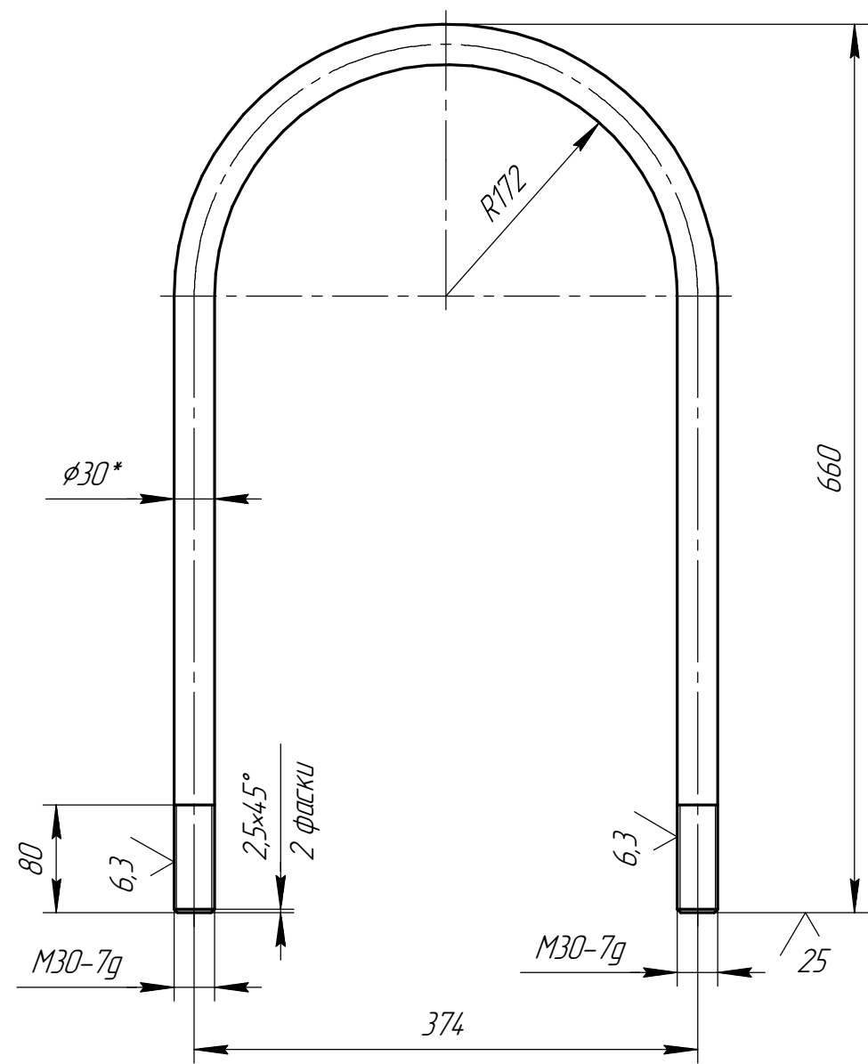
Дет. поз.2 (1:2,5)
